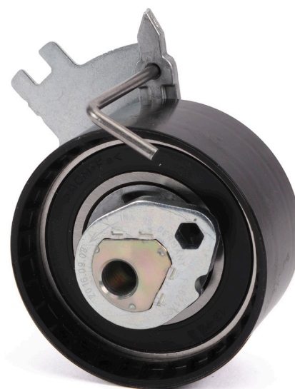
Figura 2: Rullo tenditore modificato 531 0885 10
